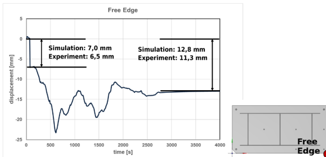
Fig. 13 Vertical deformation on free edge
